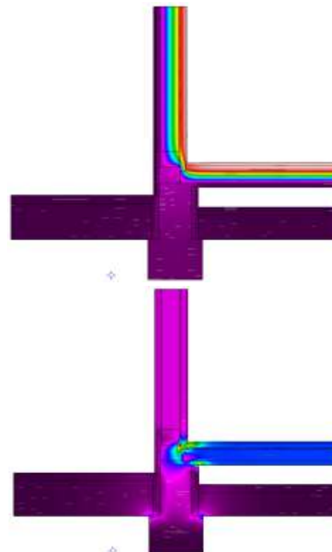
Diagramma isoterme
