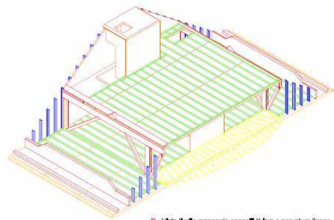
B - Vista livello mansarda pannelli X-lam e nervature linee
