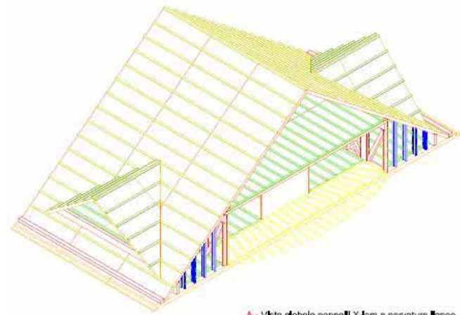
A - Vista globale pannelli X-lam e nervature linee
