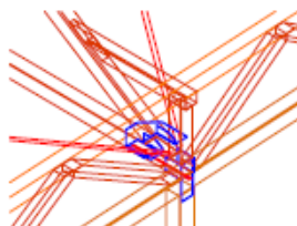
NODO PIASTRA LATO TELAIO LEGNO
