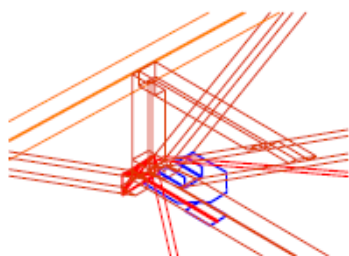
NODO PIASTRA LATO MURATURA
