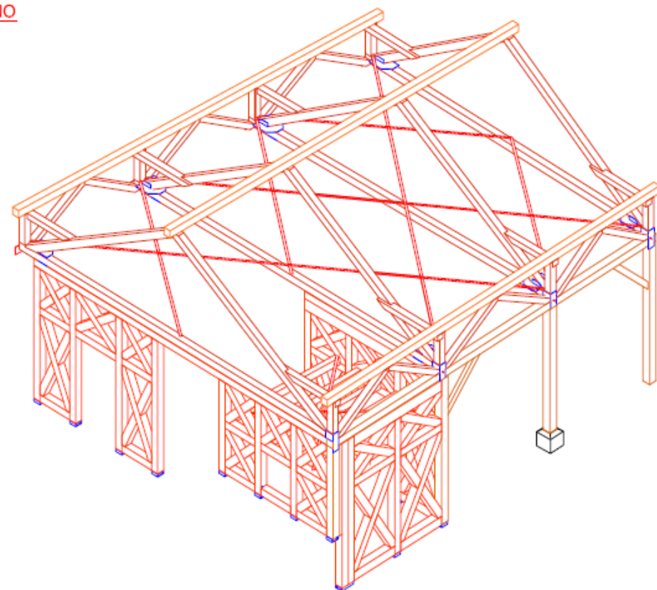
PIASTRE LATO MURATURA
