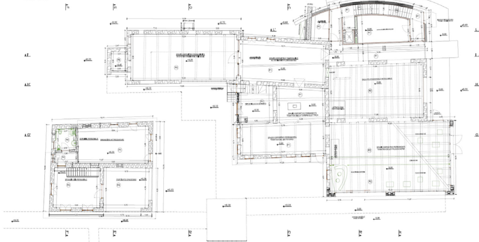
PIANTA PIANO TERRA 0 2,5 5m Scala 1:100
