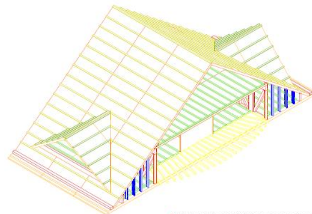
A - Vista globale pannelli X-lam e nervature linee
